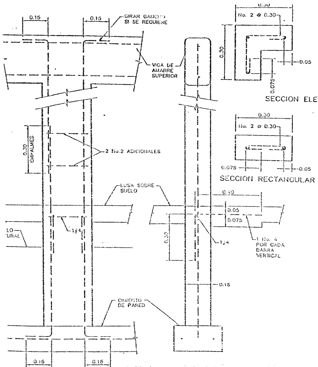
FIG. 3 DETALLES TÍPICOS DE COLUMNAS DE AMARRE
