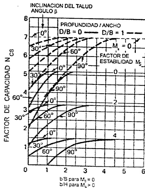
Figura 5.3.4 Capacidad de Soporte de Zapata cercana a un Talud Referencia: 9
