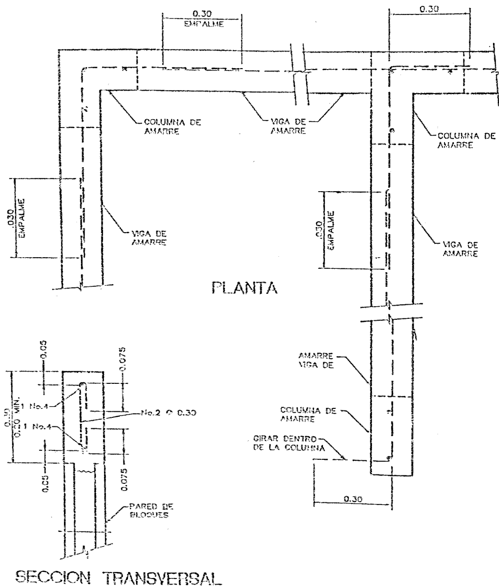
FIG. 4 DETALLES TÍPICOS DE VIGAS DE AMARRE
