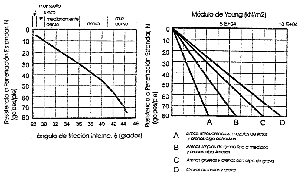
Figura 5.2.6.6 Correlación de Propiedades Mecánicas con N (SPT)
