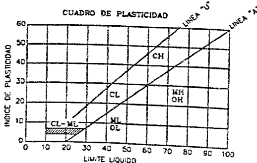
Figura 5.2.6.1 Sistema de Clasificación Unificada de Suelos Referencia(s): 5, 9, 12
