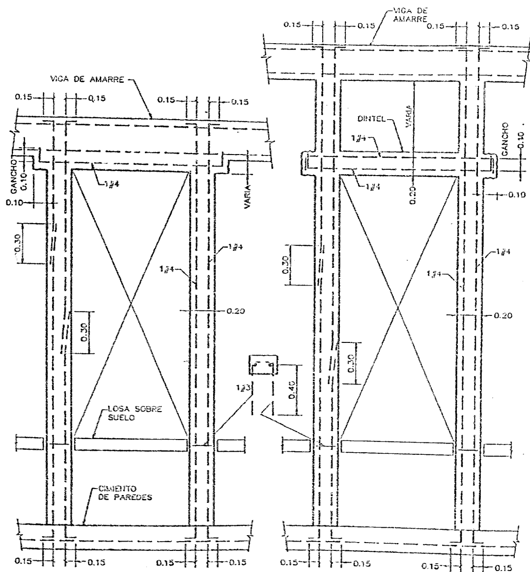
FIG. 5 REFUERZO ALREDEDOR DE PUERTAS
