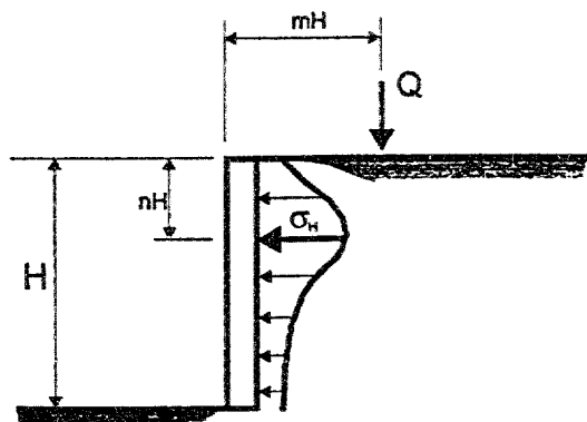
Figura 5.3.3: Presiones Laterales de Tierra
